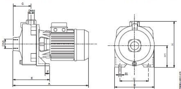
Рис. 93 NS 6-30, NS 6-40
